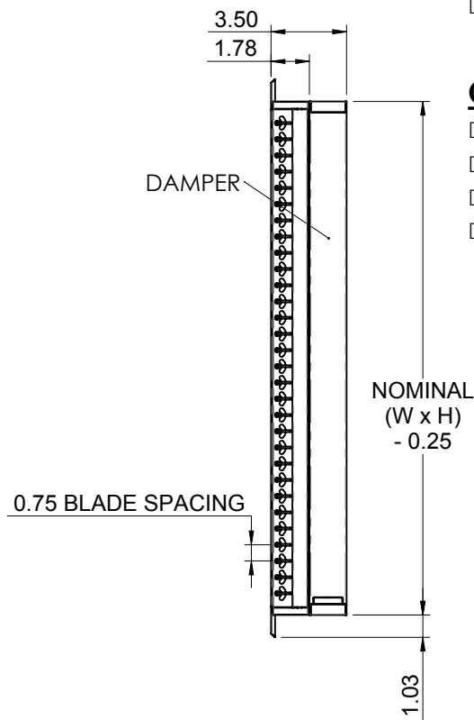
SECTION A-A
