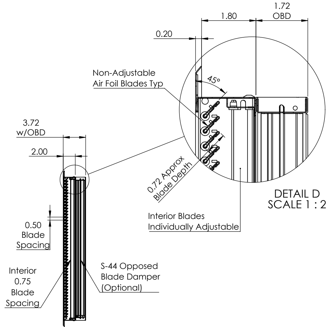
SECTION A-A
