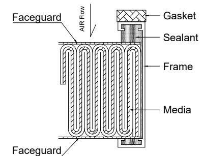
DETAIL A-A
