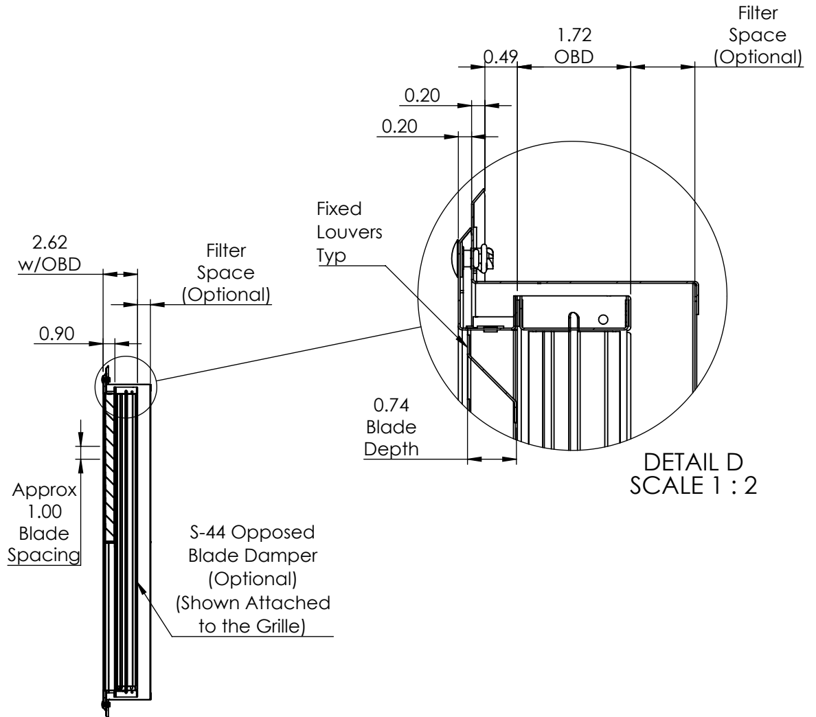
SECTION A-A
