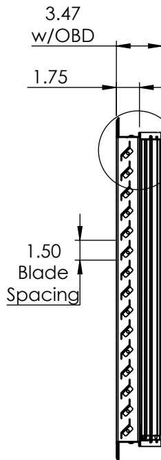
SECTION A-A
