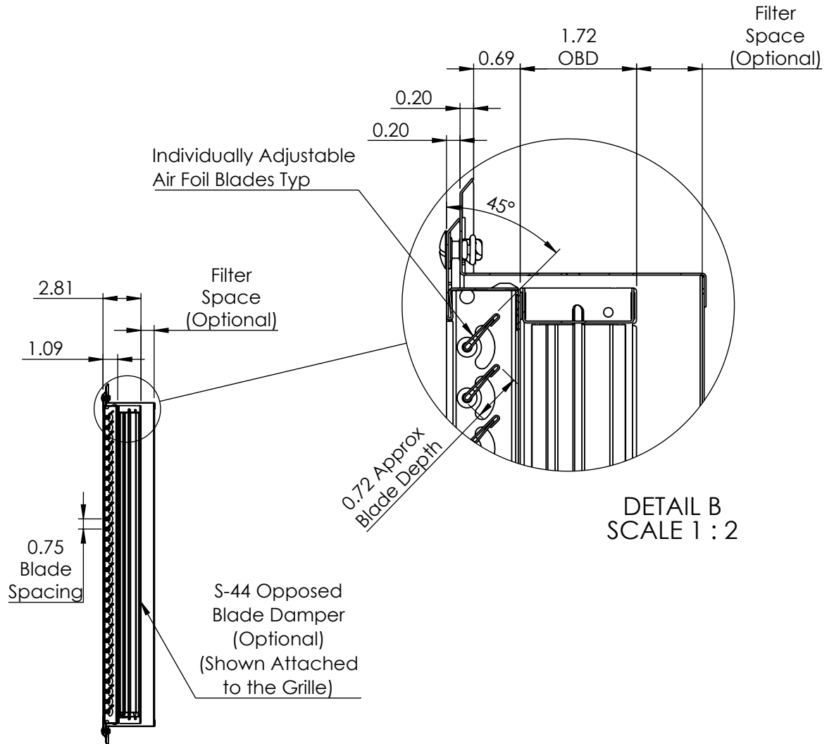
SECTION A-A
