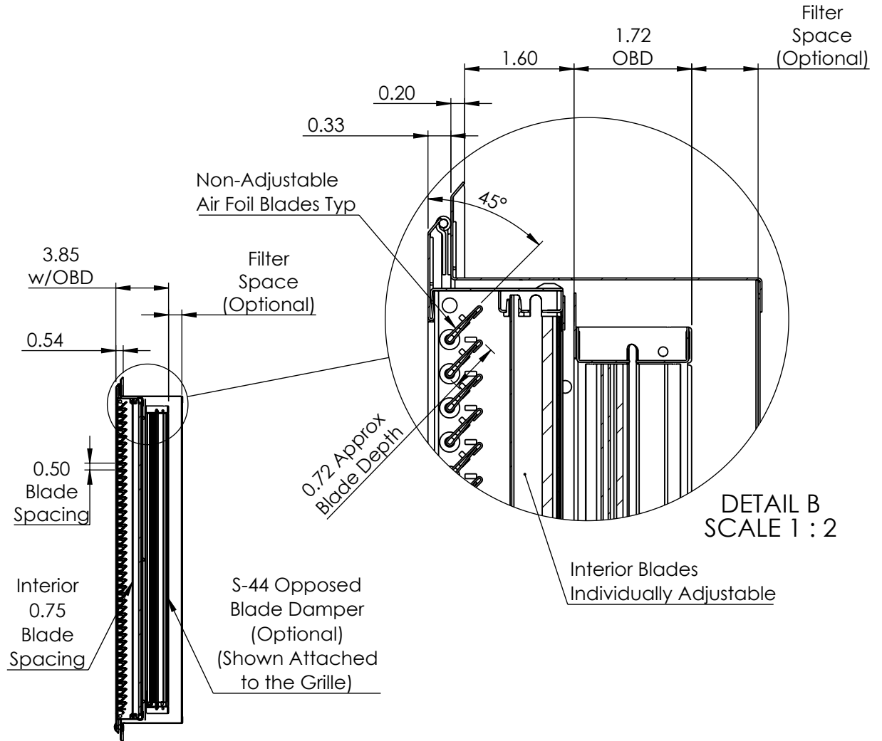
SECTION A-A
