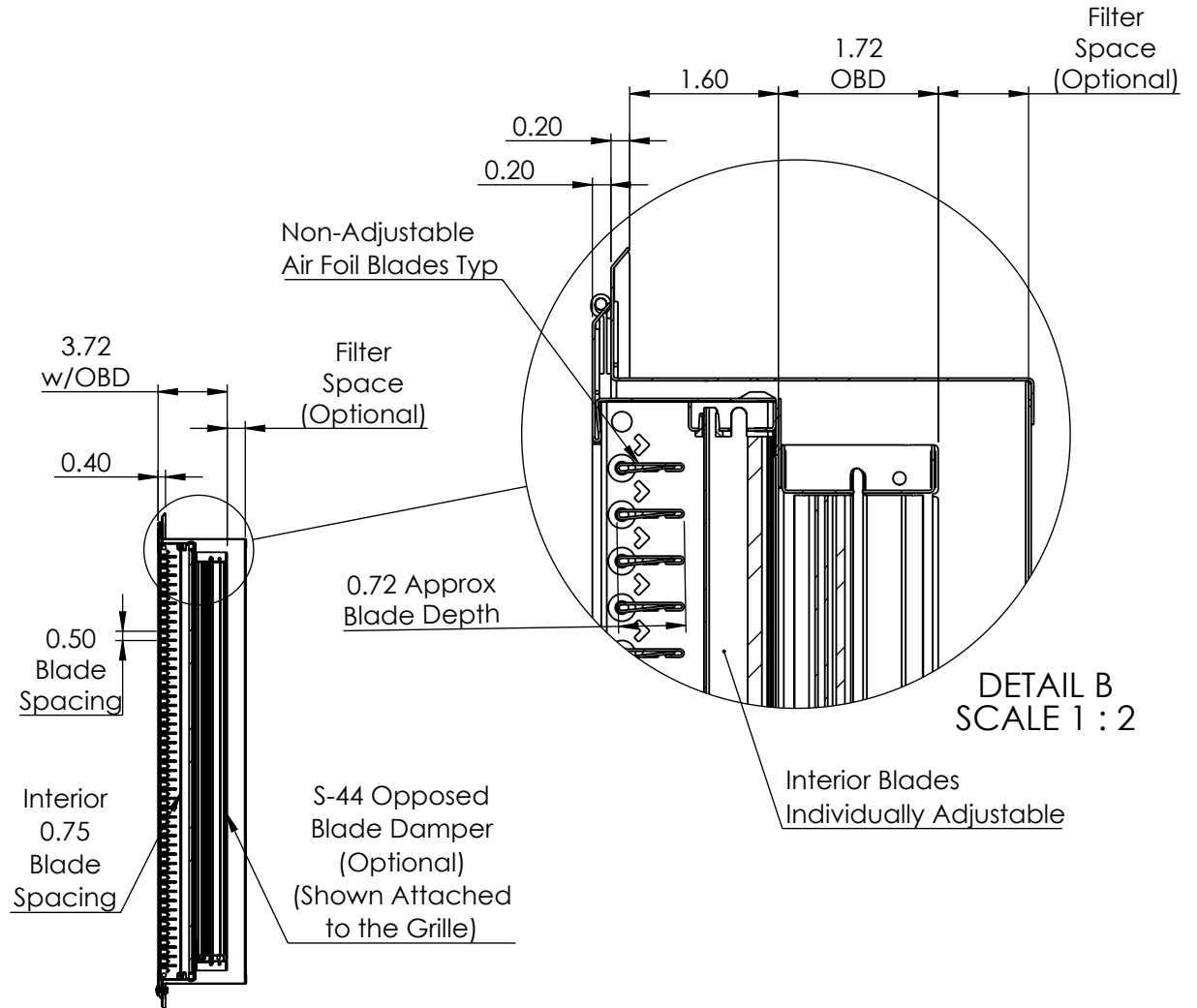
SECTION A-A
