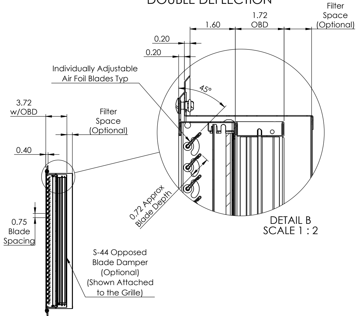
SECTION A-A
