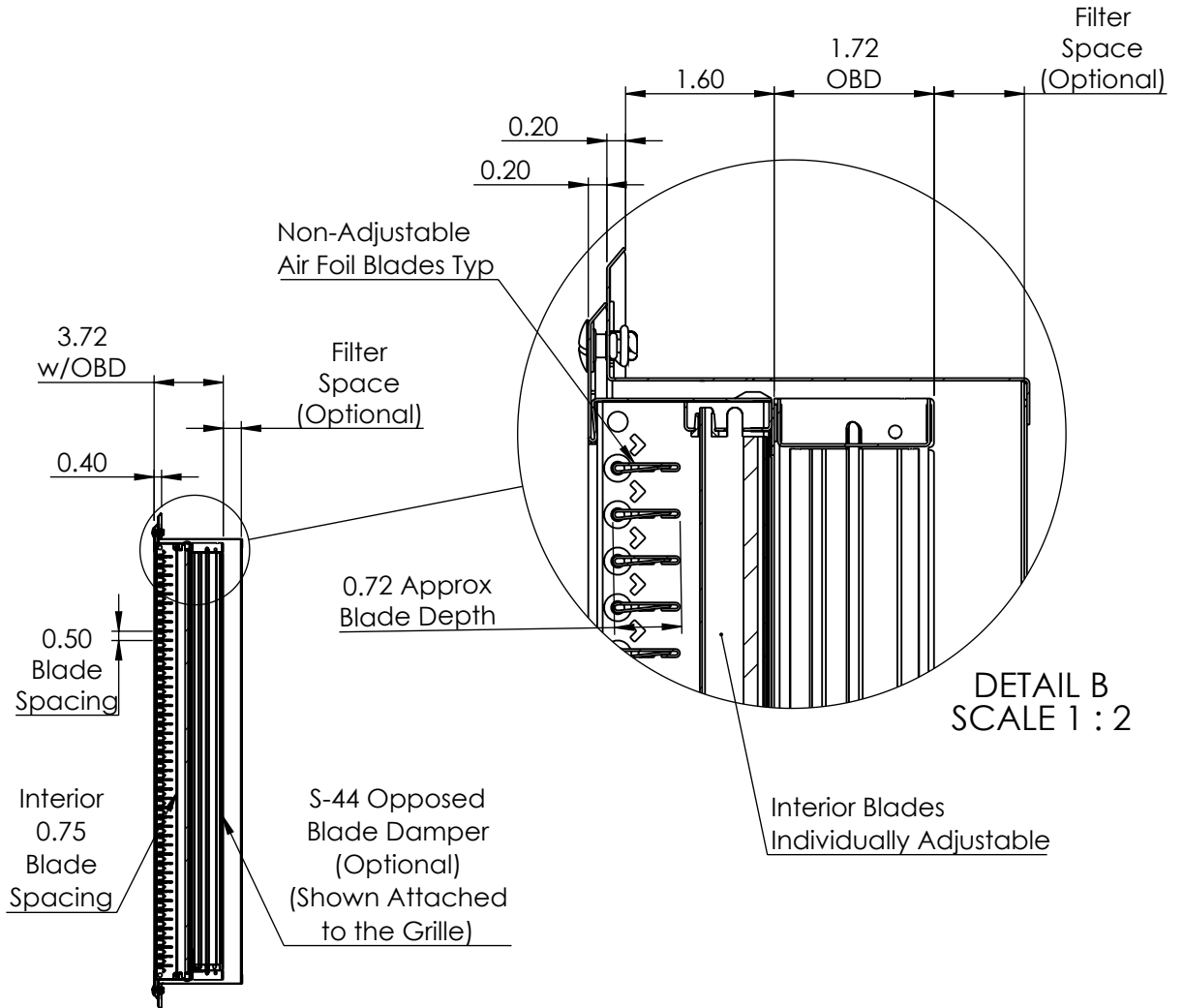
SECTION A-A
