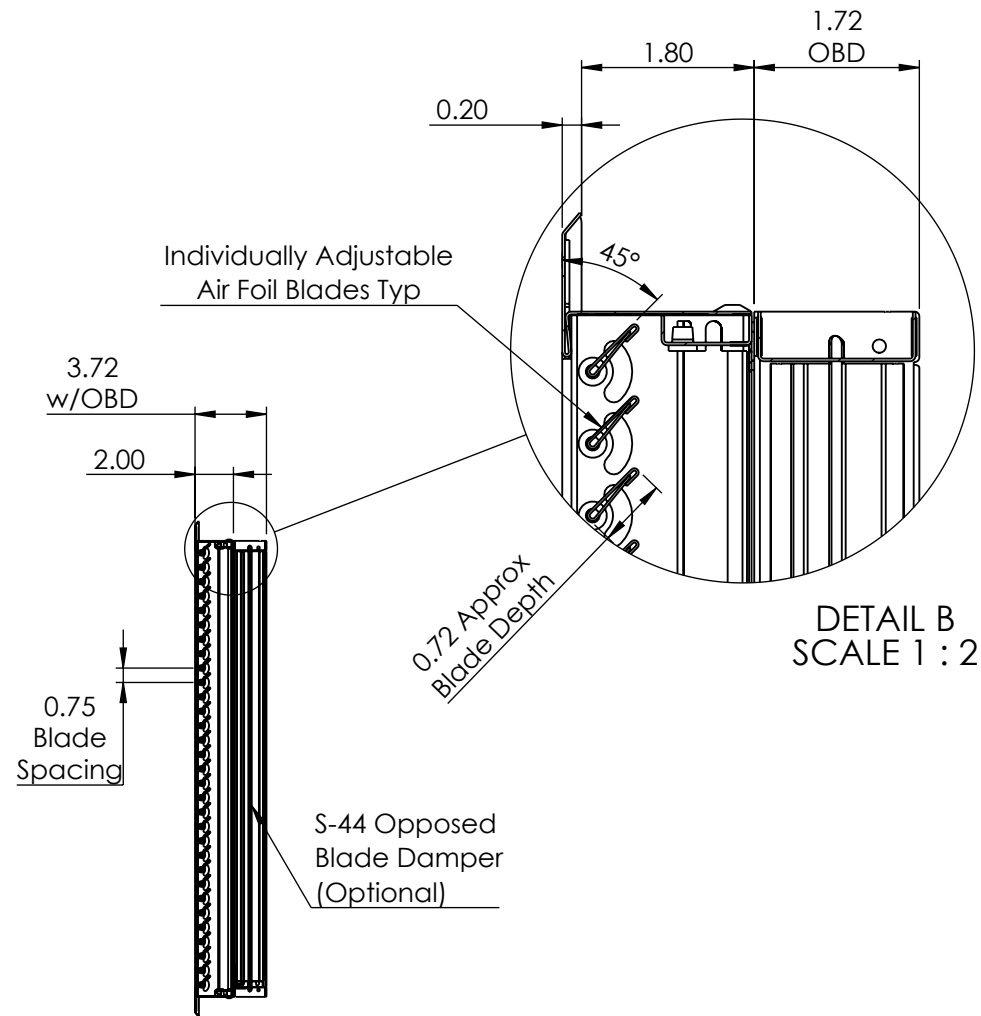
SECTION A-A
