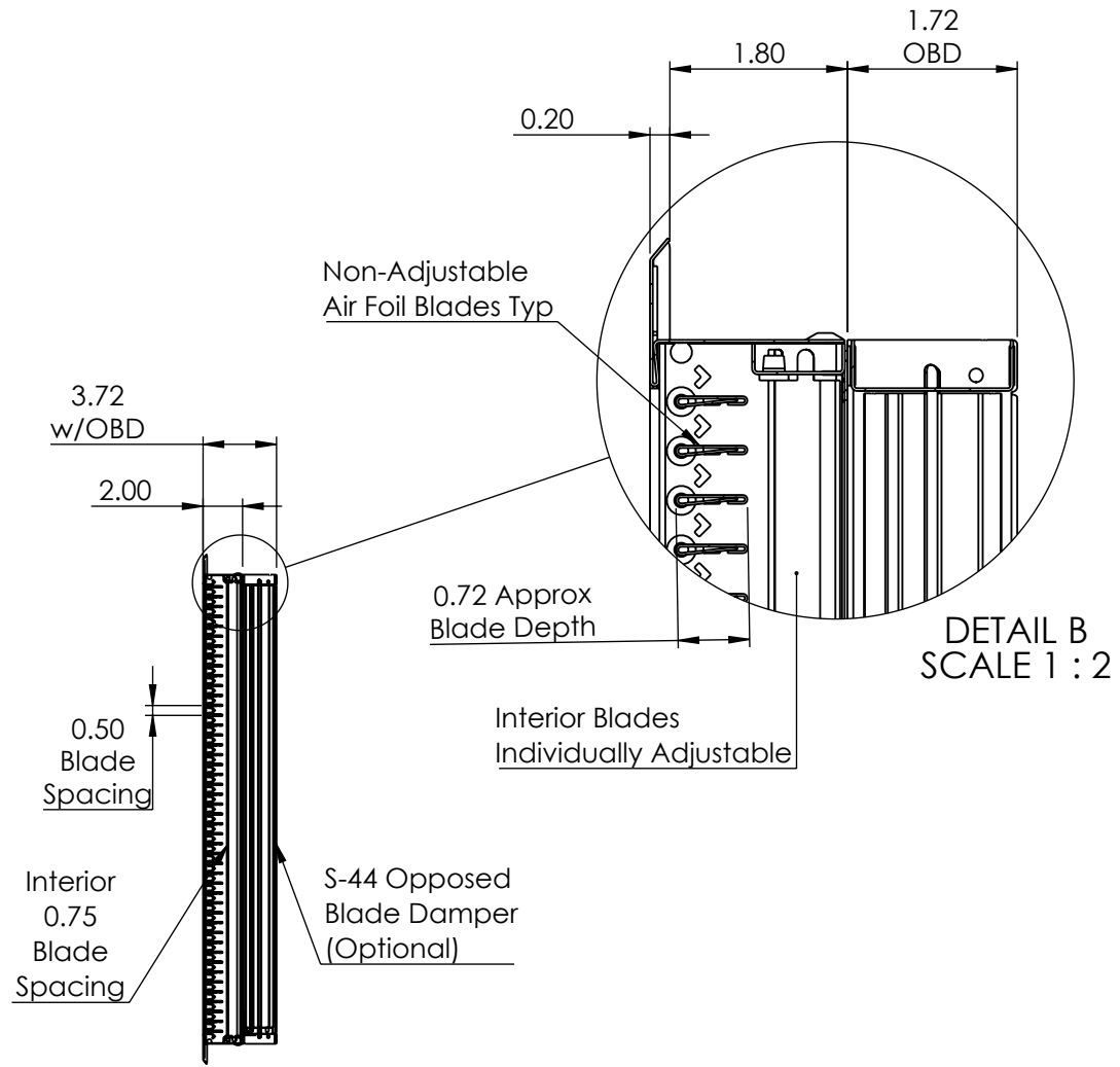
SECTION A-A
