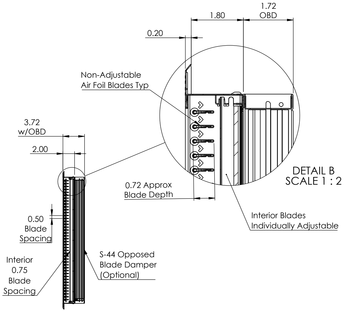
SECTION A-A
