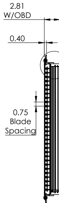
SECTION A-A
