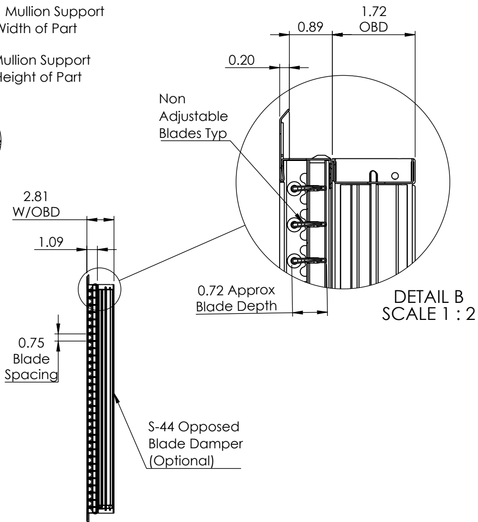
SECTION A-A
