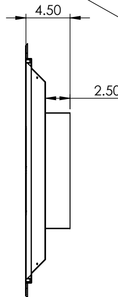
SECTION A-A
