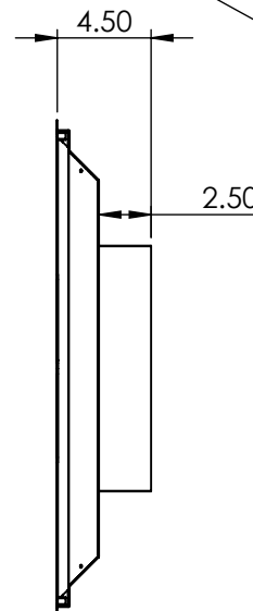
SECTION A-A
