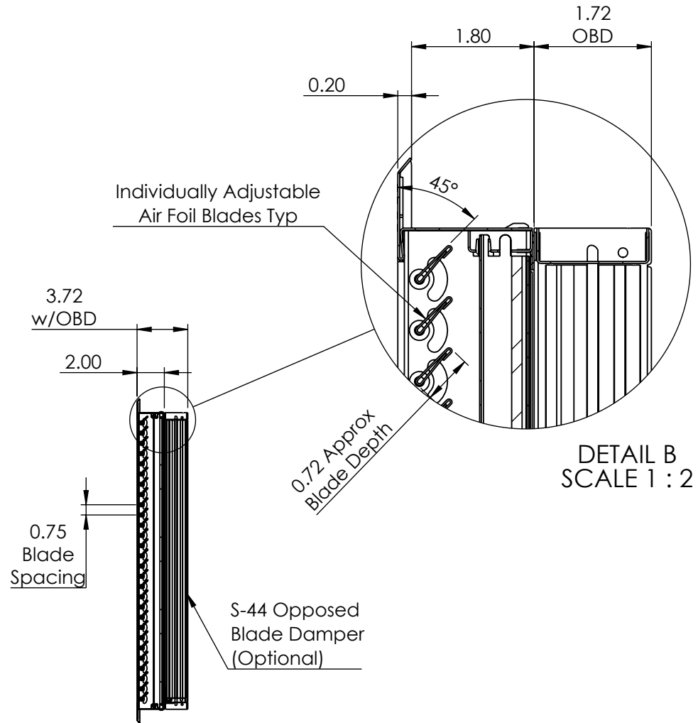
SECTION A-A
