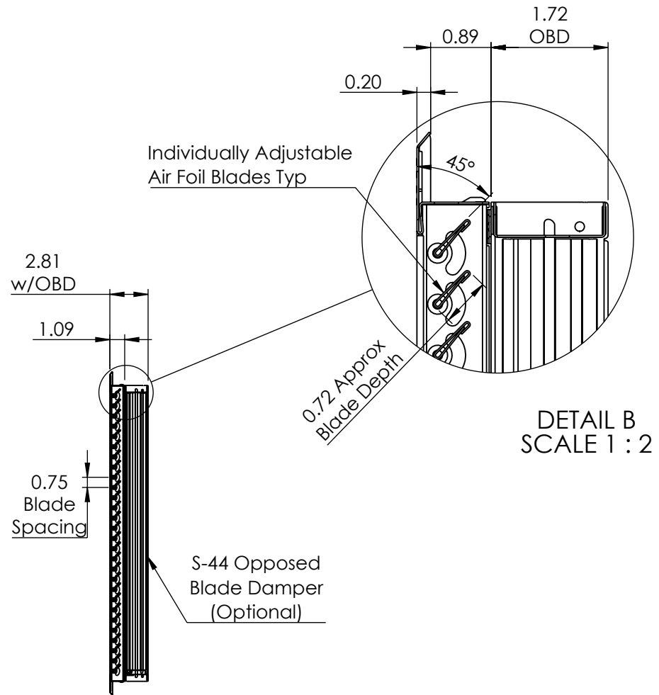
SECTION A-A
