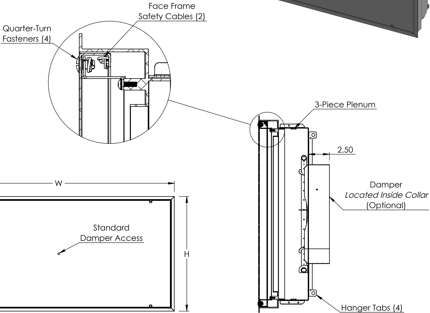
SECTION A-A SCALE 1 : 7
