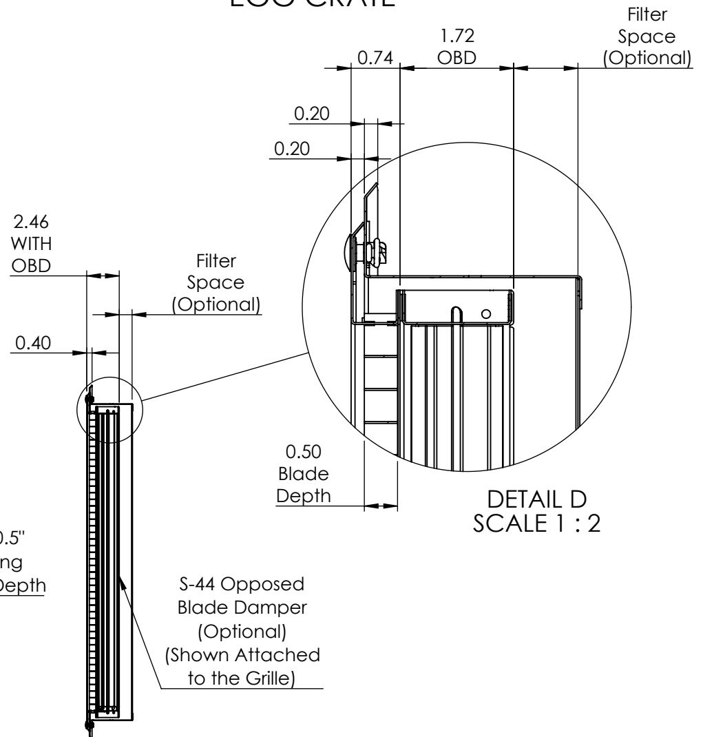
SECTION A-A
