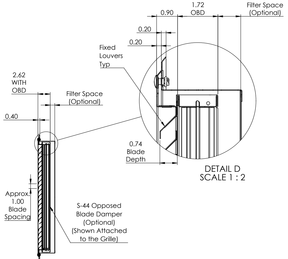
SECTION A-A
