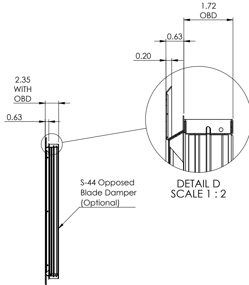
SECTION A-A
