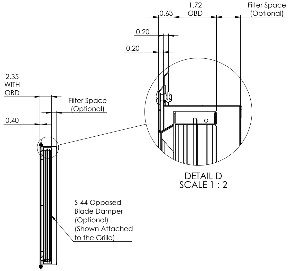
SECTION A-A
